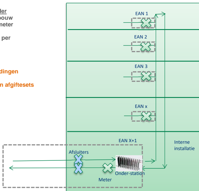
Aansluiting (koppeling op distributieleiding tot en met warmtewisselaar, inc. afsluiters & meters)
