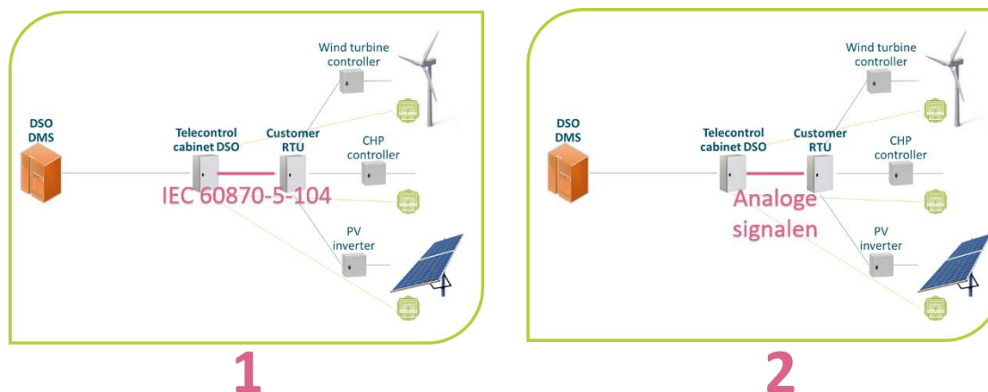
Figuur 1: Sturing via IEC 61870-5-104 of via analoge signalen.
