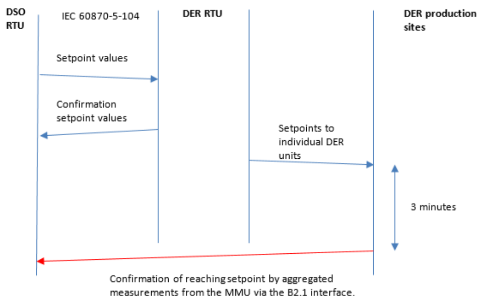
Figuur 6: Regellus via IEC 60870-5-104 en metingen.
