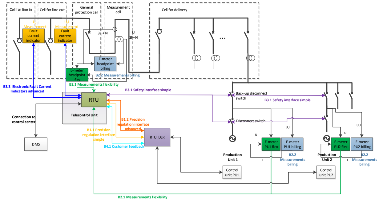
Figuur 2: Blokdiagram Ingeluste Klant
