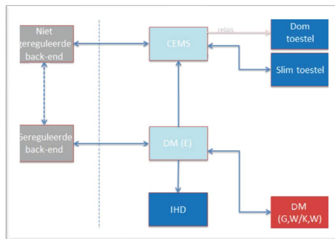
Figuur 1: Architectuur van de meetopstelling
