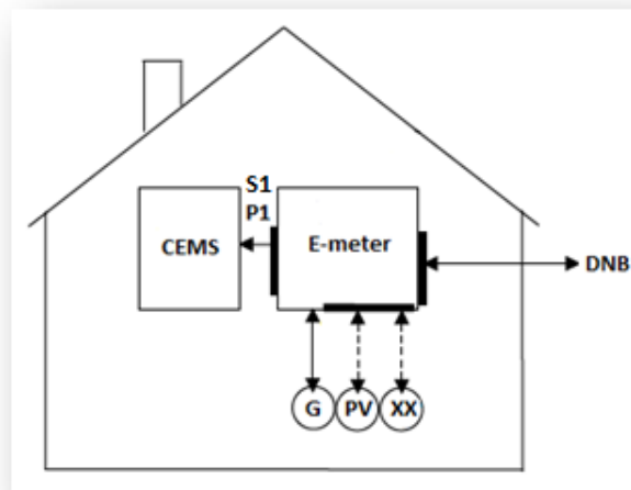
Figuur 2: Meetinrichting
