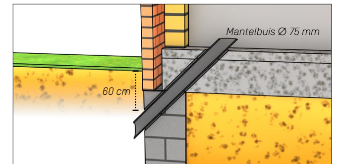
Opstelling gelijkvloers
