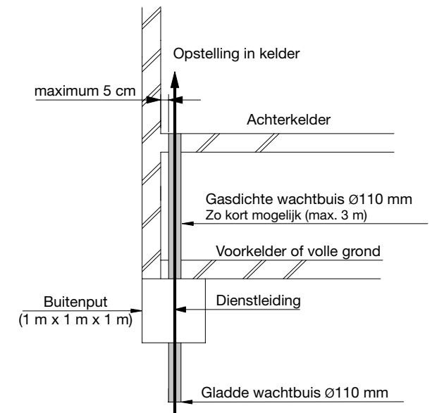
Opstelling kelder
