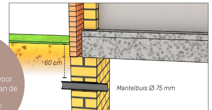
Opstelling kelder
