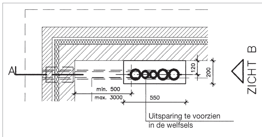
Zijaanzicht
