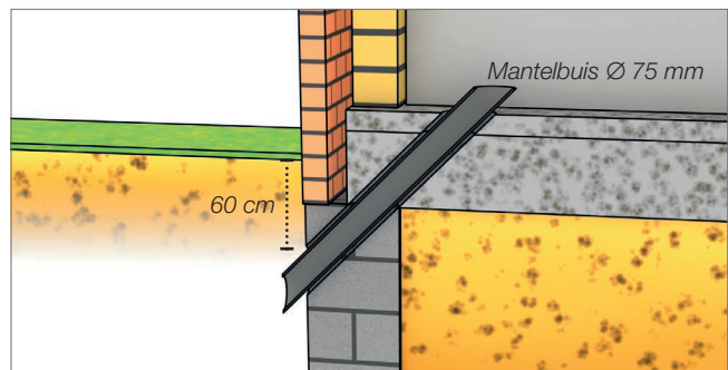
Opstelling gelijkvloers
